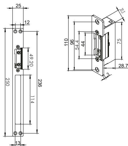
DIMENSÕES PARA EMBUTIR O FECHO NO BATENTE
