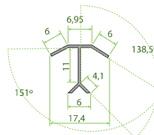
CANTONEIRA SEXTAVADA
